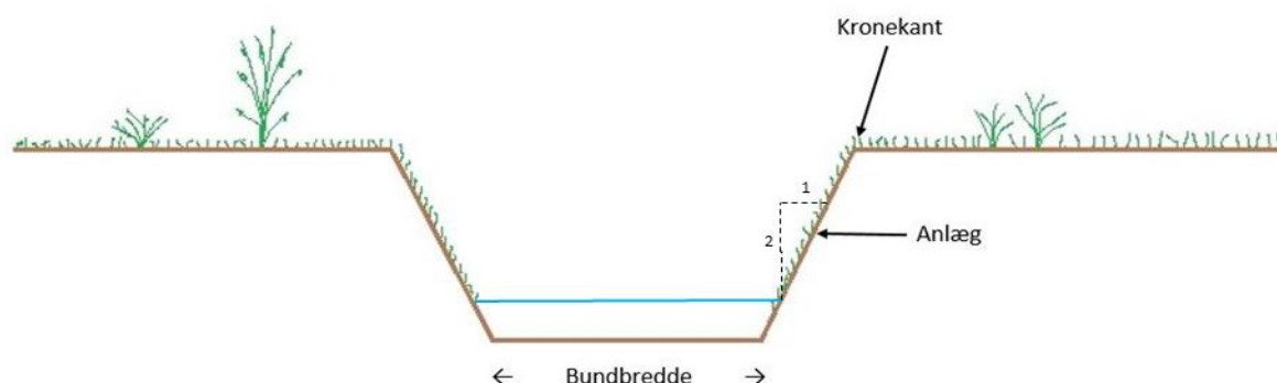
Figur 1-2 Principtegning til illustration af de i regulativet angivne betegnelser. Vandløbets skråning skaldes også for brinken.
