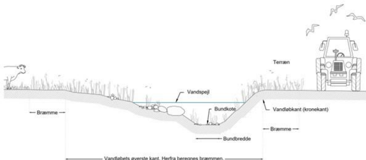
Figur 1-3 Illustration af vandløbsprofil og 2-meter bræmmen.
